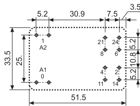
Ansicht auf die Anschlüsse
